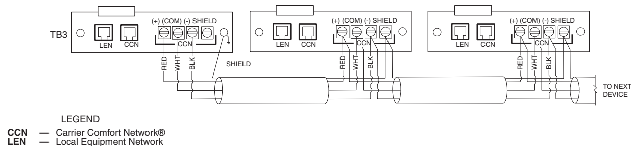
Fig. 62 — TB-3 — CCN Wiring
